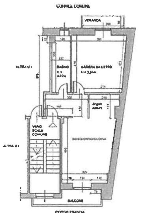
PLANIMETRIA INDICATIVA STATO ATTUALE - fuori scala
