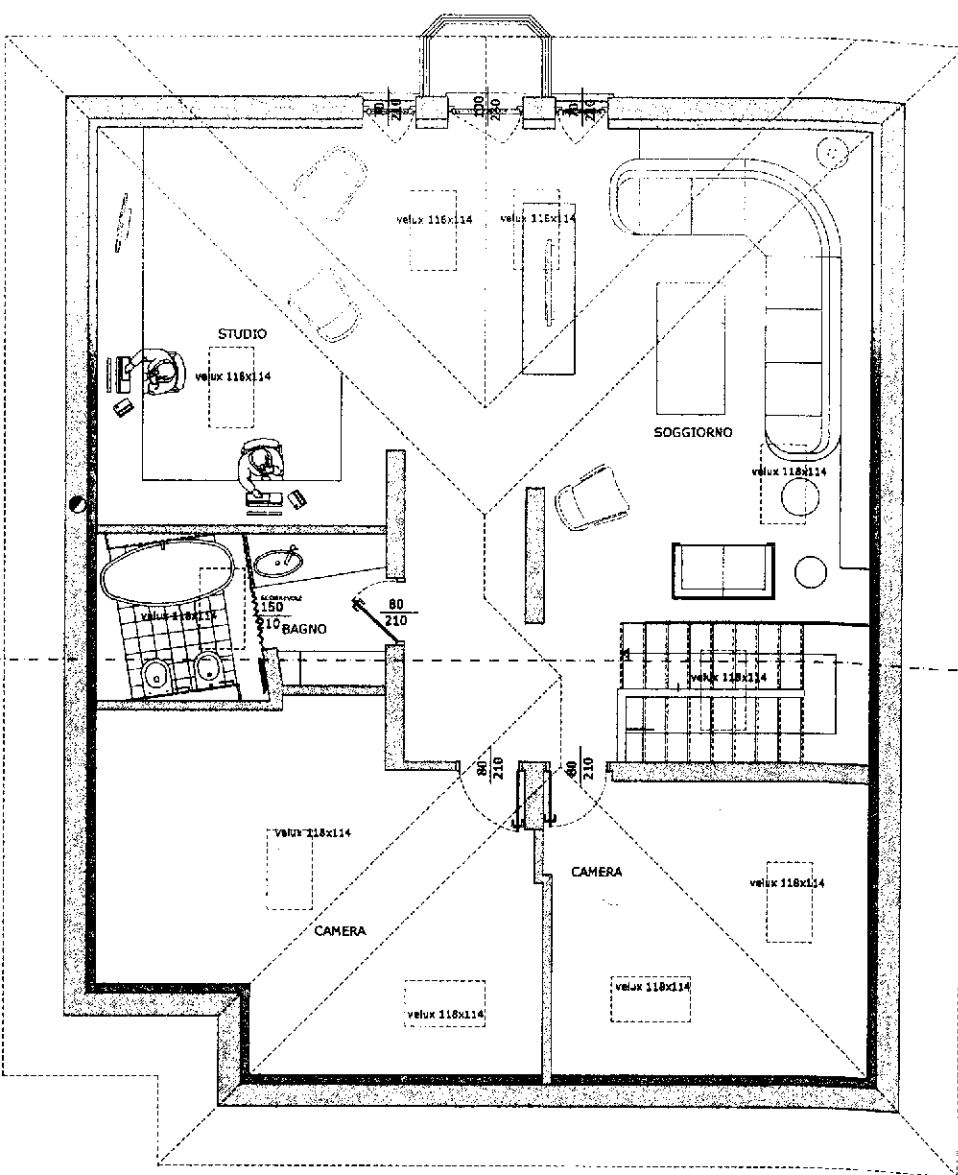
SOTTOTETTO
