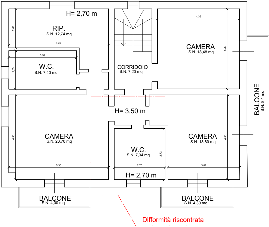
PIANO PRIMO
