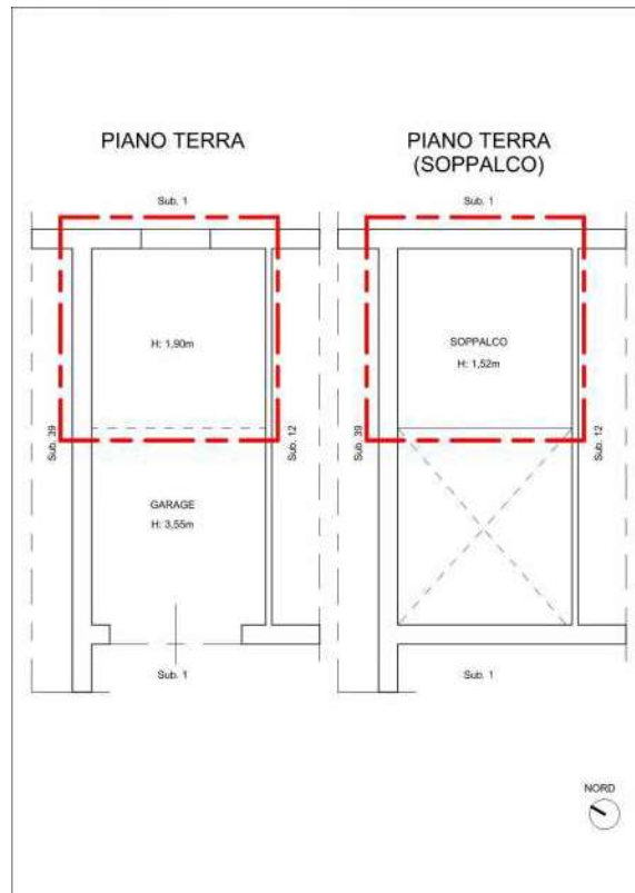
Pianta piano terra (Immobile n.2) - Plan. Stato reale
