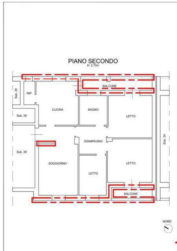
Piano Piano Secondo - Plan. Stato reale
